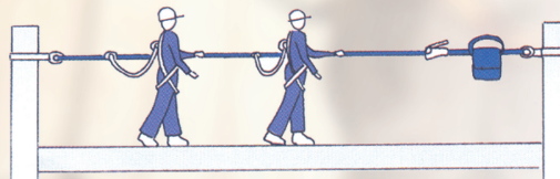
梳織扁帶橫定向式安全裝置 Ref. : 1012060 (便攜安全裝置) Ref. : 1012113 (連 2 條固定吊裝帶)
